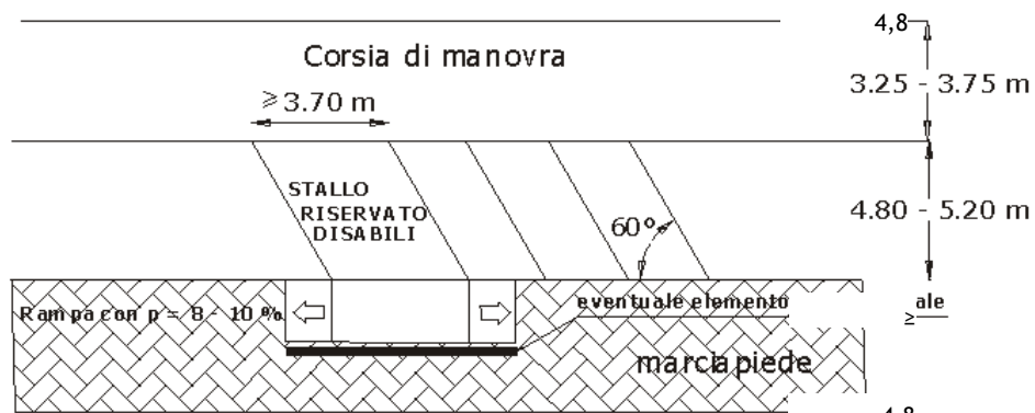
Stalli di sosta a spina
