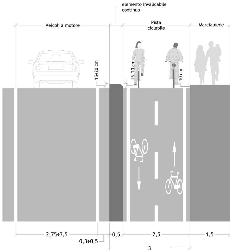
Figura 2 Sezione tipo: Pista ciclabile in sede propria - separazione invalicabile
