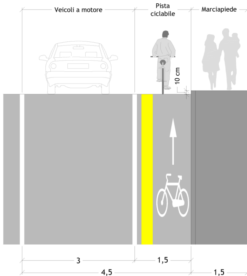
Figura 5 Sezione tipo: Pista ciclabile su corsia riservata su carreggiata monodirezionale
