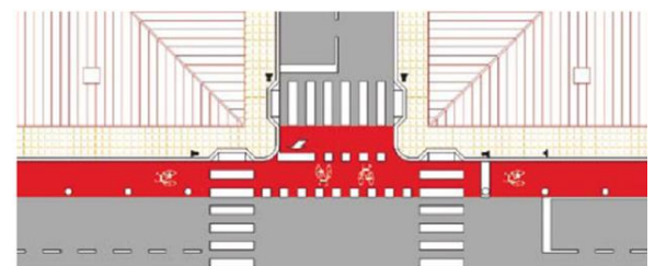
ESEMPI DI SVOLTA A SINISTRA INDIRETTA
