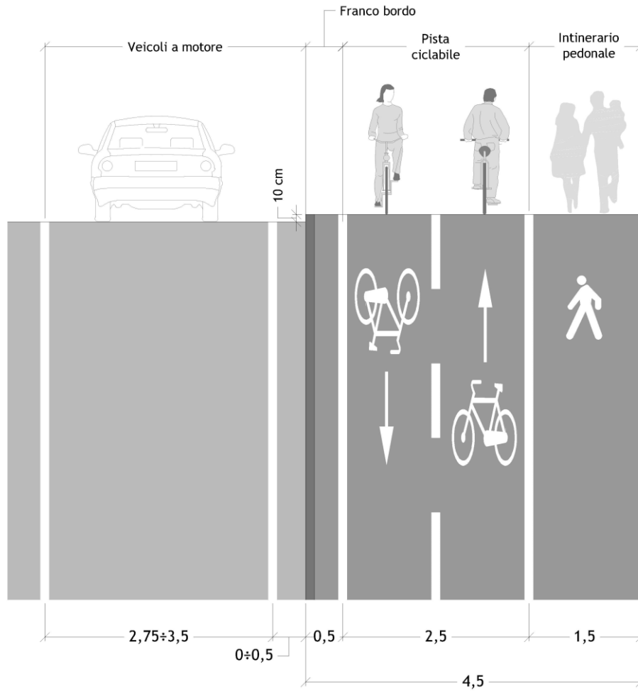
Figura 9 Sezione tipo: Pista ciclabile su corsia riservata sui marciapiedi
