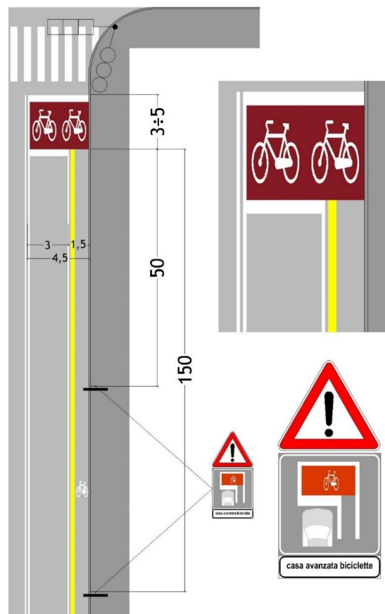
Figura 33 Schemi planimetrici di Casa avanzata per le biciclette
