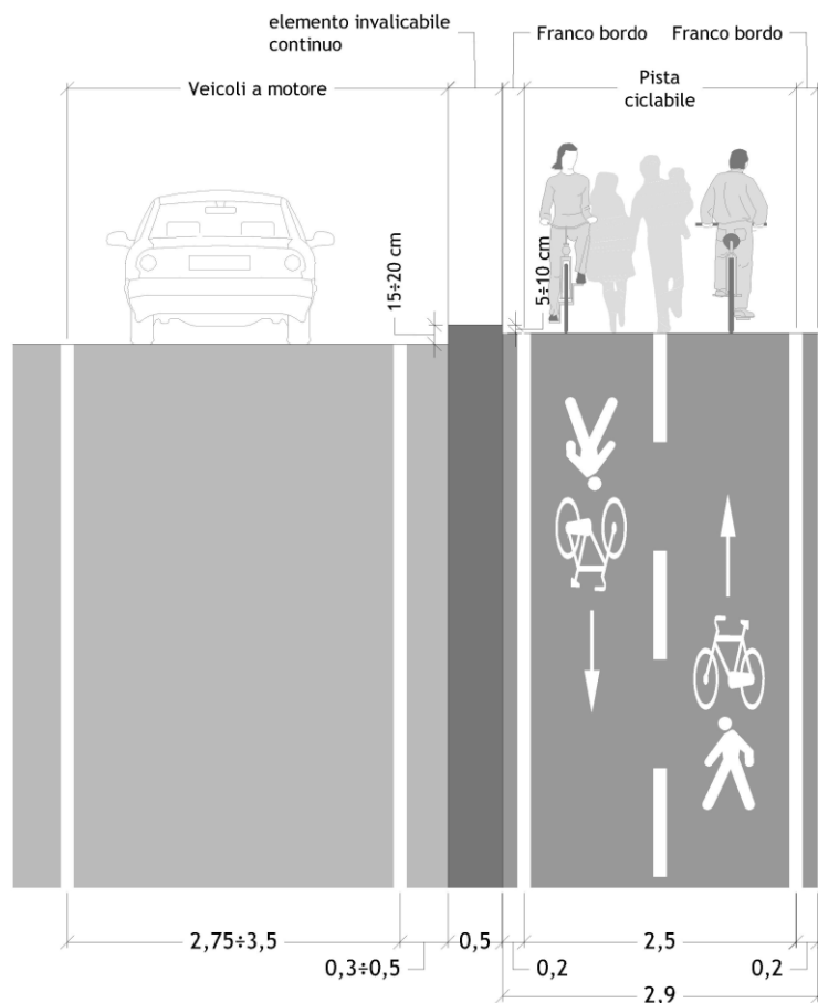
Figura 28 Sezione tipo: Percorsi promiscui pedonali e ciclabili
