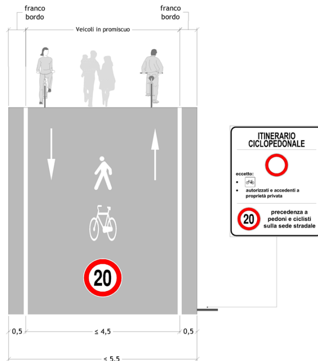
Figura 24 Sezione tipo: Strada F-Bis
