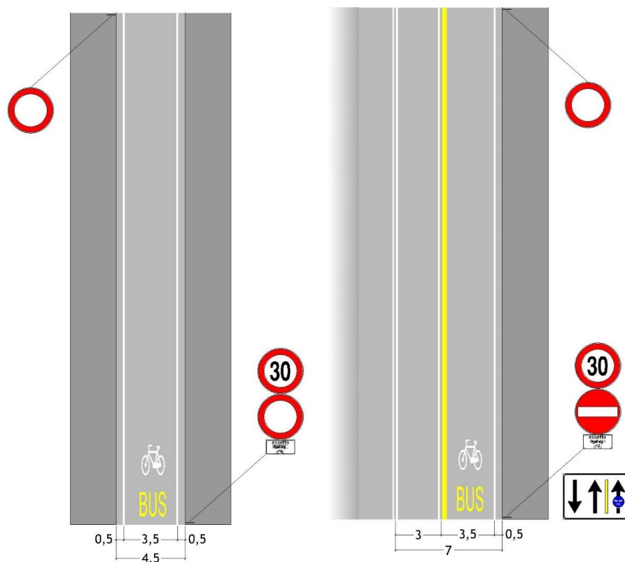
Figura 34 Schemi planimetrici di Flusso ciclabile nella corsia riservata al trasporto pubblico locale
