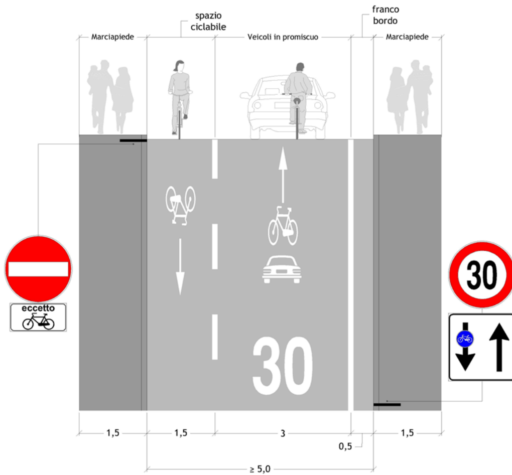
Figura 17 Sezione tipo: Corsie ciclabili per doppio senso ciclabile
