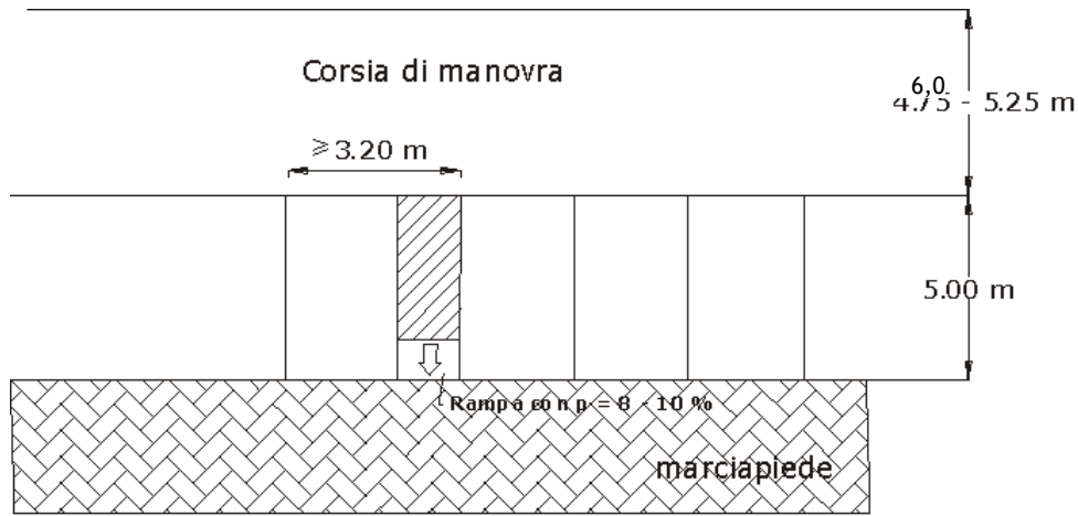
Stalli di sosta a pettine
